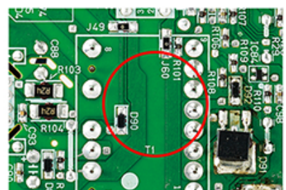
主機板AC高電壓/ DC低電壓採隔離設計
