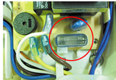
主機板電流保險絲
