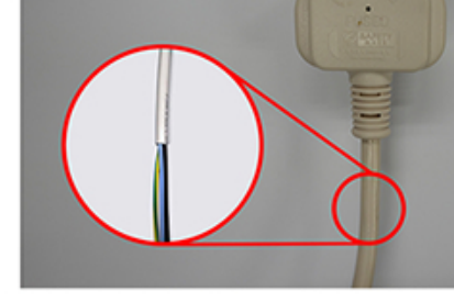
雙重絕緣電源線
