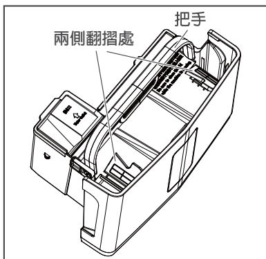
水箱蓋拆下方法
